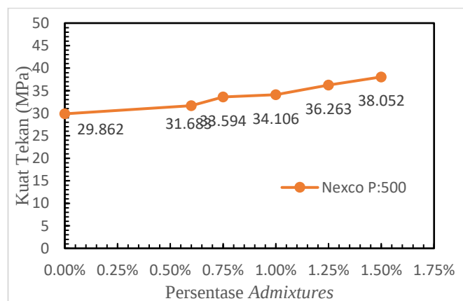
Gambar 6. Hasil uji kuat tekan beton dengan admixture Nexco Polynex He 500.
