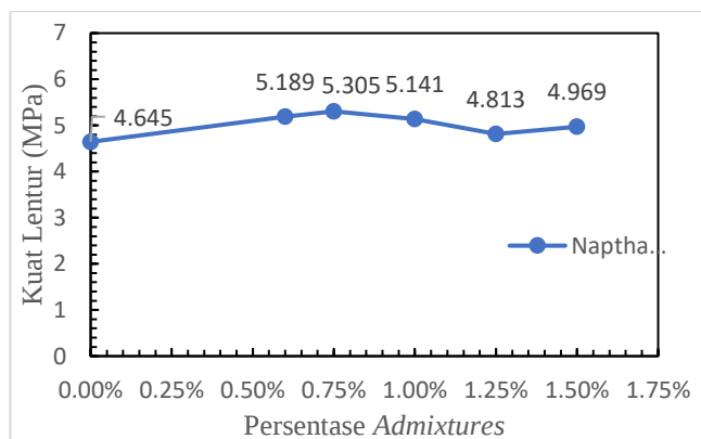
Gambar 8. Grafik hasil uji kuat lentur beton dengan admixtures Naptha E121.
