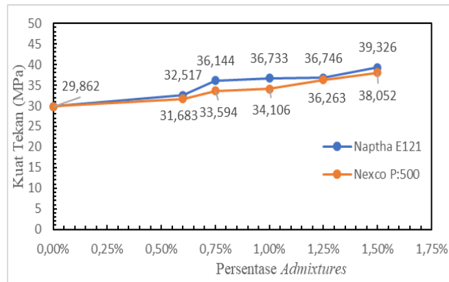
Gambar 7. Grafik perbandingan kuat tekan beton dengan admixture Naptha E121 dan Nexco Polynex He 500.
