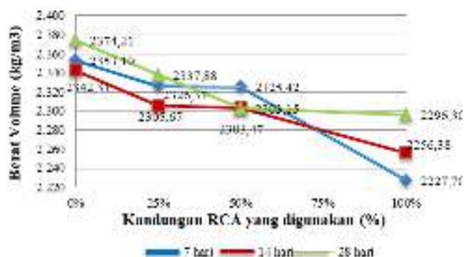
Gambar 3. Hubungan berat volume beton dengan variasi penggantian sebagian agregat kasar dengan RCA
